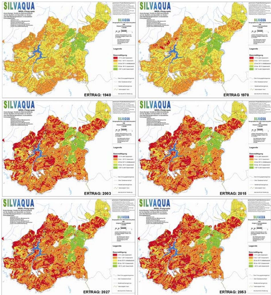
Abbildung 5: Modellerte räumliche und zeitliche Dynamik der Basensättigung im Wurzelraum für das Waldentwicklungsszenario ERTRAG (Legende: ■: < 5 %, ■: 5 bis < 20 %, ■: 20 bis < 50 %, ■: 50 bis < 80 %, ■: > 80 % Basensättigung)
