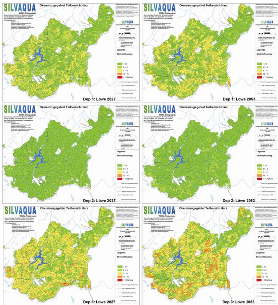
Abbildung 4: Modellerte N-Auswaschung mit dem Sickerwasser für das Waldentwicklungsszenario LÖWE bei veränderten N-Depositionen (■: < 2,5, ■: 2,5 bis < 5, ■: 5 bis < 10, ■: 10 bis < 15, ■: > 15 kg·ha -1 ·a -1 . Dep1 = BAS, Dep2 = GOT und Dep3 = HIG, vgl. auch Tabelle 2)
