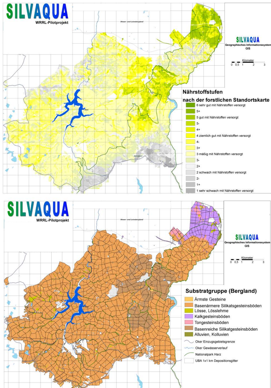
Abbildung 5: Die Nährstoffstufen (oben) und Substratgruppen (unten) nach der niedersächsischen forstlichen Standortskartierung im Okereinzugsgebiet „Teilbereich Nordharz“
