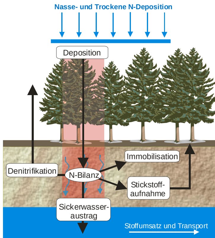
Abbildung 1: Schematische Darstellung der einbezogenen Bilanzgrößen des Stickstoffkreislaufes
