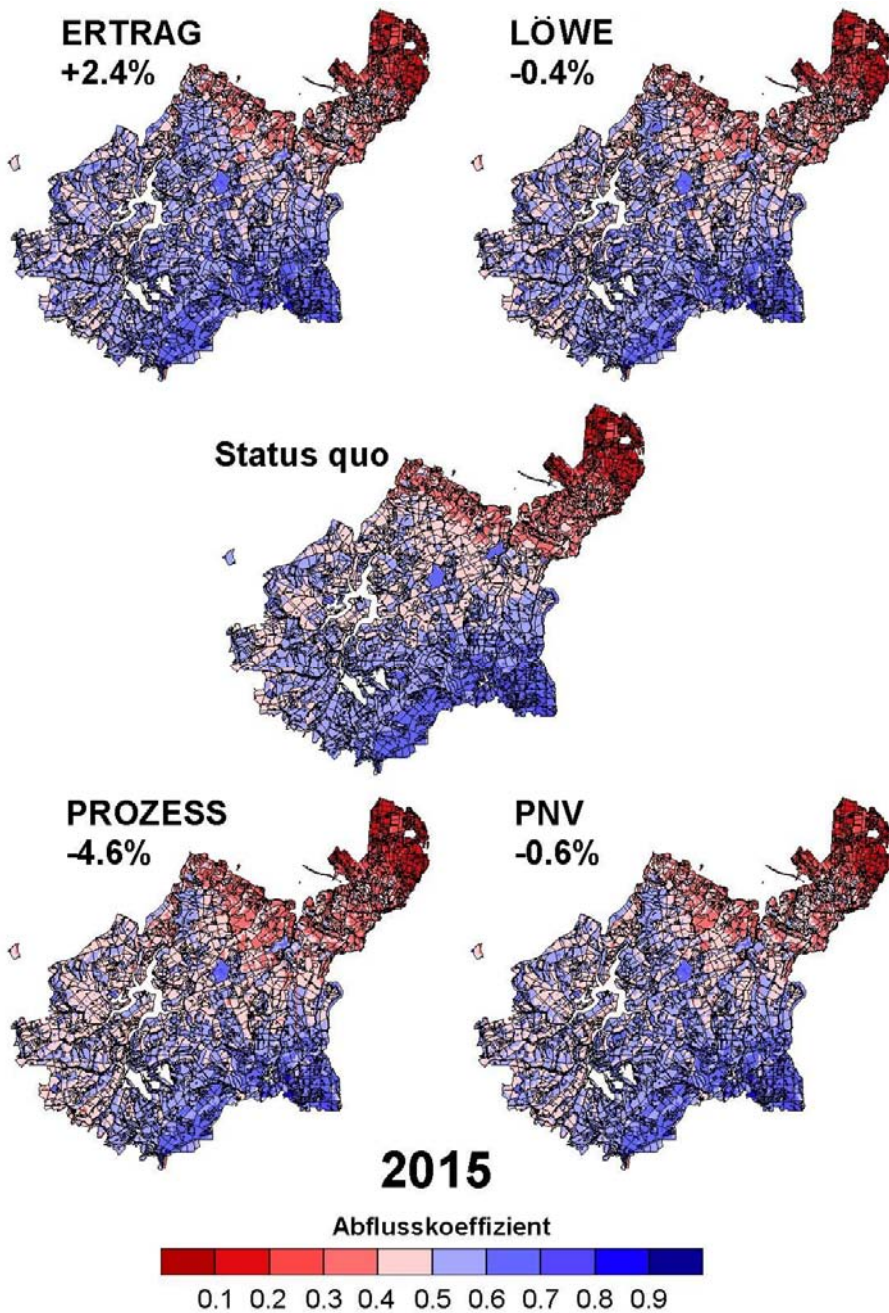
Abbildung 5: Berechnete Abflusskoeffizienten für die Waldentwicklungsszenarien im Zeitfenster 2015
