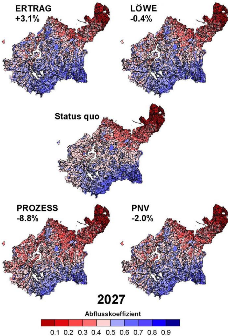
Abbildung 6: Berechnete Abflusskoeffizienten für die Waldentwicklungsszenarien im Zeitfenster 2027
