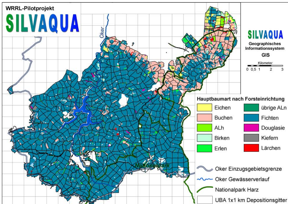
Abbildung 9: Räumliche Verteilung der Hauptbaumarten gemäß der Forsteinrichtung von 2003
