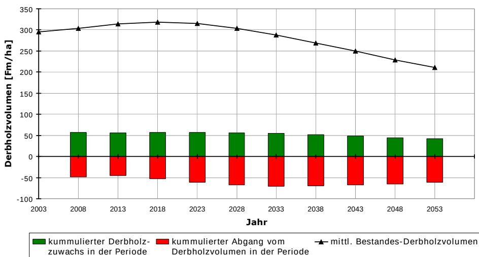
Abbildung 4: Dynamik des mittleren Bestandes-Derbholzvolumens für das Szenario LÖWE (flächen-gewichtetes Mittel aller Waldbestände des Untersuchungsgebietes)
