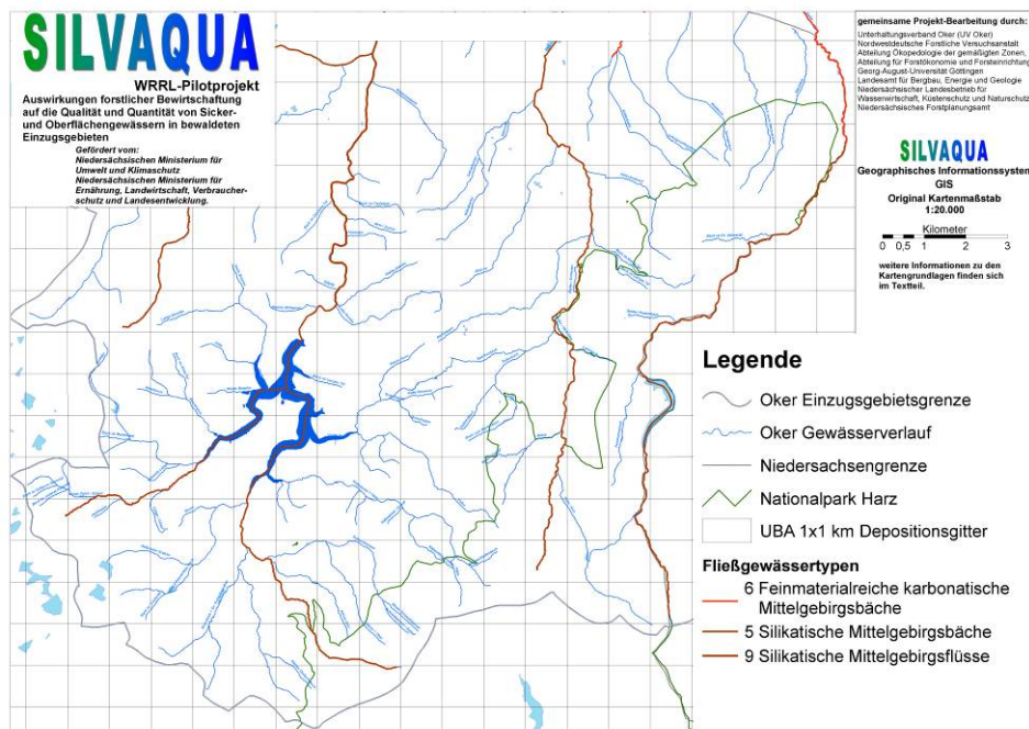
Abbildung 6: Fließgewässertypen im Okereinzugsgebiet „Teilbereich Nordharz“. Für die blau eingezeichneten Gewässer liegen keine Daten zum Gewässertyp und zur Qualität vor.
