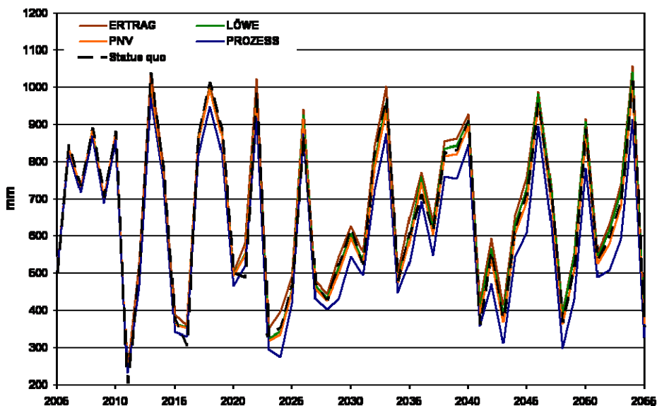
Abbildung 4: Berechneter Abfluss [mm] für die Waldentwicklungsszenarien
