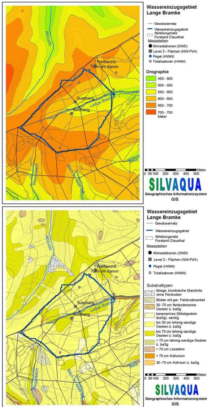
Abbildung 11: Orographie und Substrattypen im Teileinzugsgebiet der „Lange Bramke“
