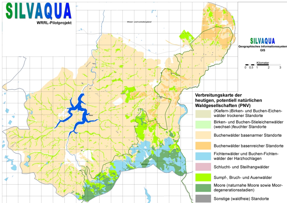
Abbildung 3: Heutige potenziell natürliche Waldgesellschaften im Okereinzugsgebiet „Teilbereich Nordharz“
