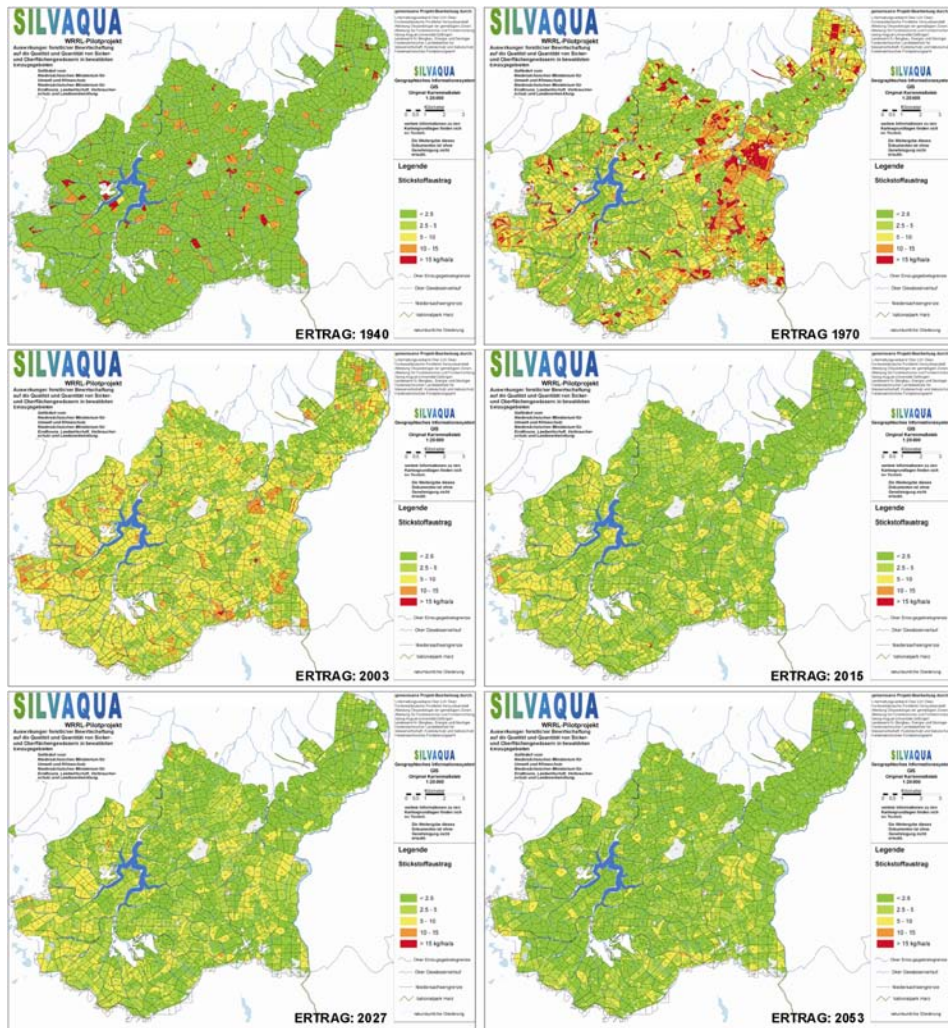
Abbildung 2: Modellerte räumliche und zeitliche Dynamik der Stickstoffauswaschung mit dem Sickerwasser für das Waldentwicklungsszenario ERTRAG (■: < 2,5, ■: 2,5 bis < 5, ■: 5 bis < 10, ■: 10 bis < 15, ■: > 15 kg·ha -1 ·a -1 )
