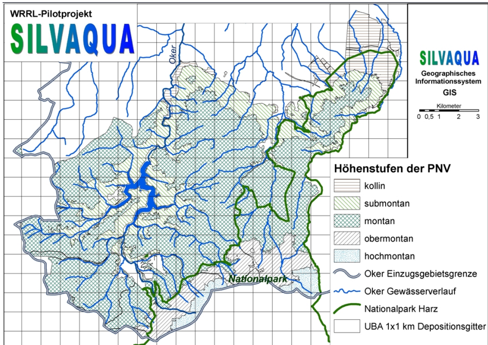
Abbildung 2: Höhenstufen für die Zuordnung der PNV im Okereinzugsgebiet „Teilbereich Nordharz“ mit dem zusätzlich eingezeichneten Gewässernetz
