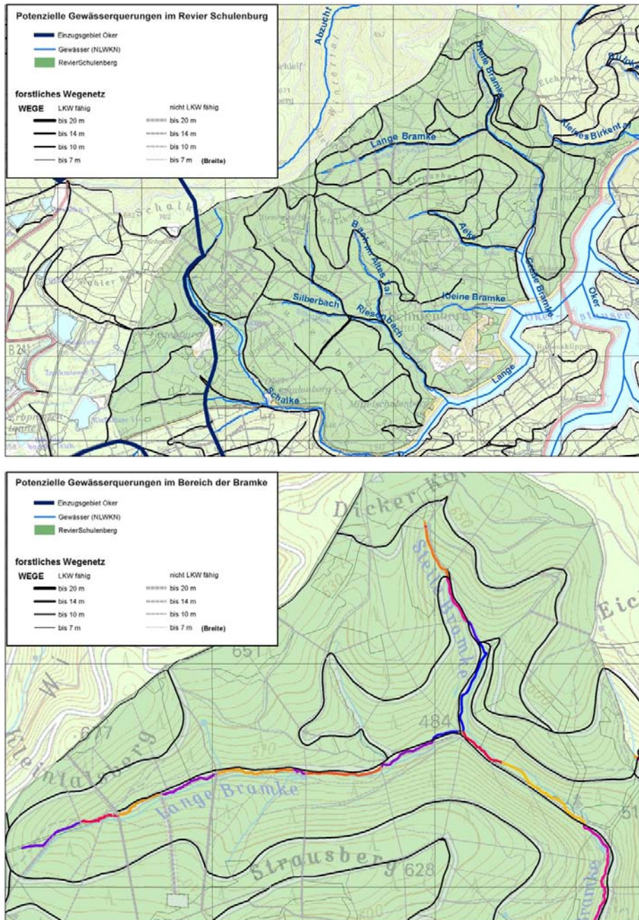
Abbildung 5: Potenzielle Gewässerquerungen durch das forstliche Wegenetz im Revier Schulenburg im Bereich der „Bramke“; einzelne Gewässerabschnitte sind im farblichen Wechsel hervorgehoben
