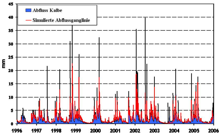
Abbildung 2: Gemessene und simulierte Abflussganglinie am Pegel Kalbe
