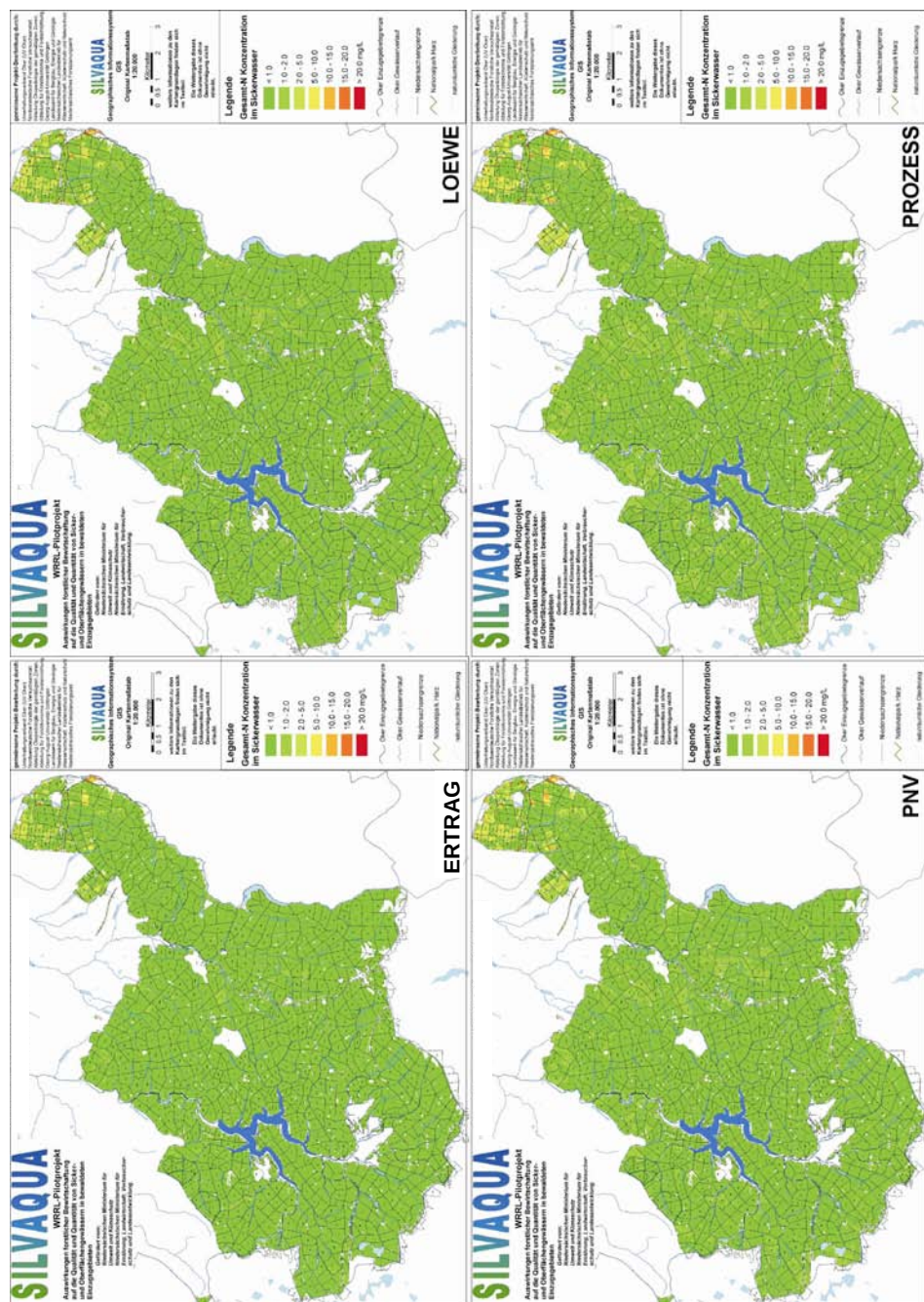
Abbildung 7: Mittlere \text{NO}_3 -Konzentrationen für die Waldentwicklungsszenarien im Zeitraum von 2030 bis 2049 (■: < 1, ■: 1 bis < 2, ■: 2 bis < 5, ■: 5 bis < 10, ■: 10 bis < 15, ■: 15 bis < 20, ■: > 20 mg/l)
