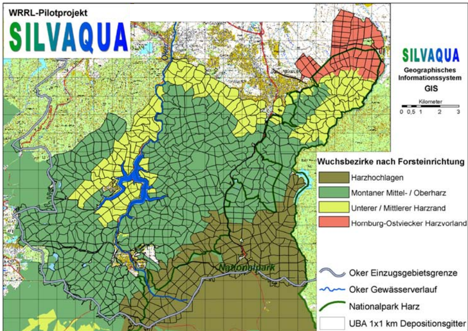
Abbildung 7: Forstliche Wuchsbezirke im Okereinzugsgebiet „Teilbereich Nordharz“ (nach Forsteinrichtungsdaten)
