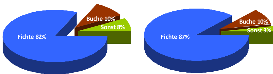
Abbildung 8: Flächenanteile (links) und Derbolzvolumenanteile (rechts) der Baumarten im Untersuchungsgebiet „Nordharz“
