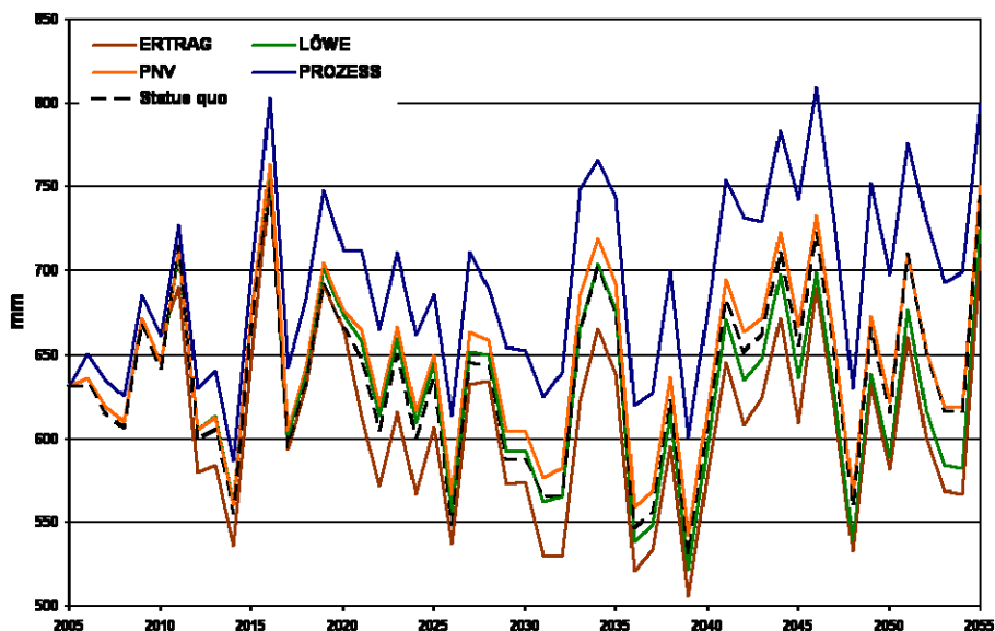
Abbildung 3: Berechnete reale Verdunstung [mm] für die Waldentwicklungsszenarien
