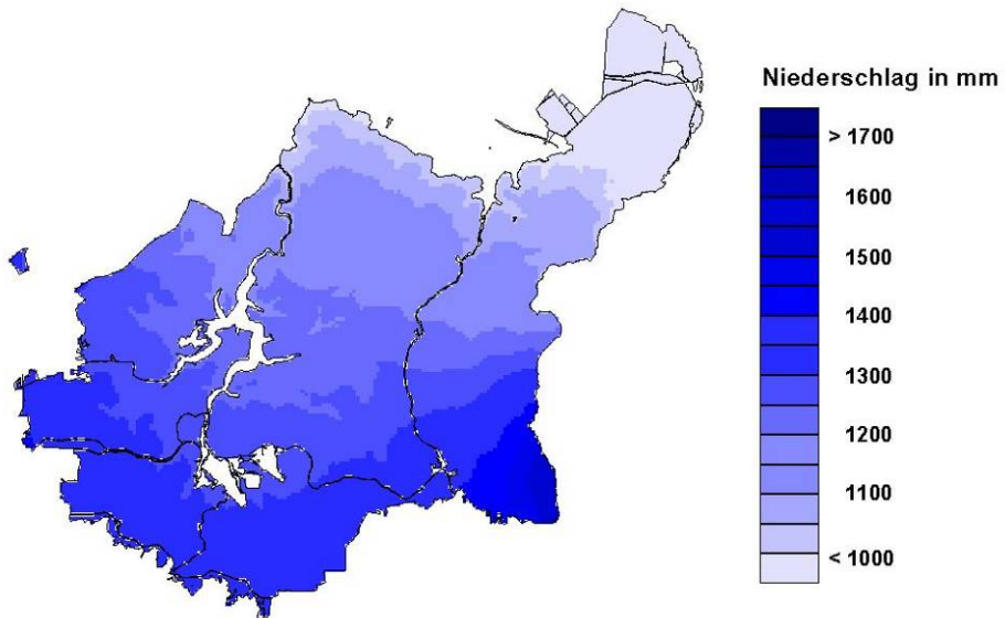
Abbildung 2: Niederschlagsverteilung im Untersuchungsgebiet (mittlere Jahressumme 1996 - 2005)
