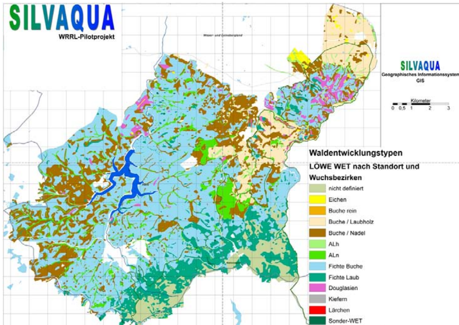
Abbildung 1: Waldentwicklungstypen nach den aktuellen LÖWE-Richtlinien zur Baumartenwahl (NIEDERSÄCHSISCHE LANDESFORSTVERWALTUNG 2004) im Okereinzugsgebiet „Teilbereich Nordharz“
