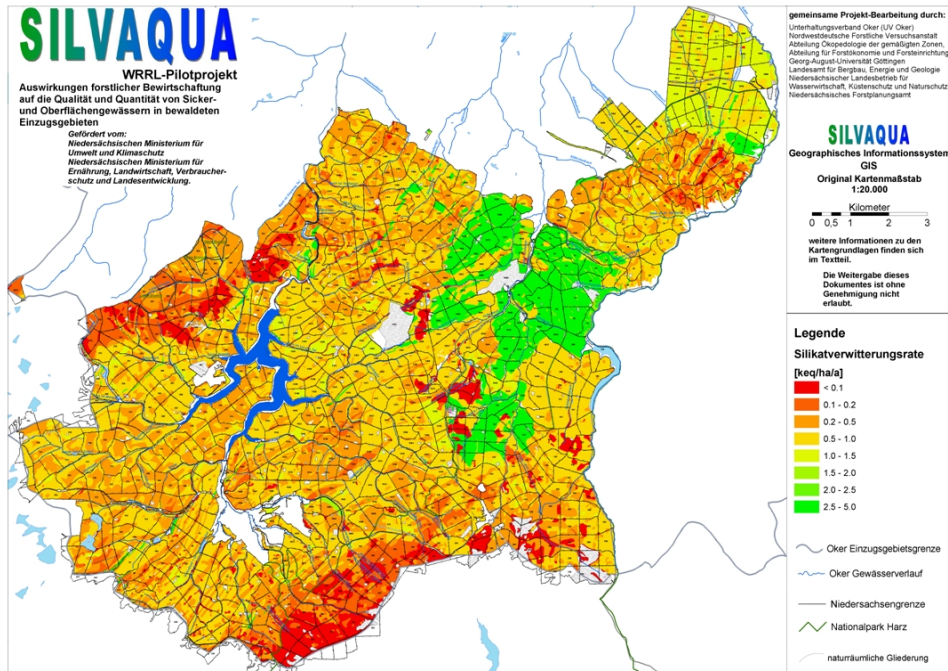
Abbildung 2: Regionalisierung der Silikatverwitterungsraten im Okereinzugsgebiet „Teilbereich Nordharz“
