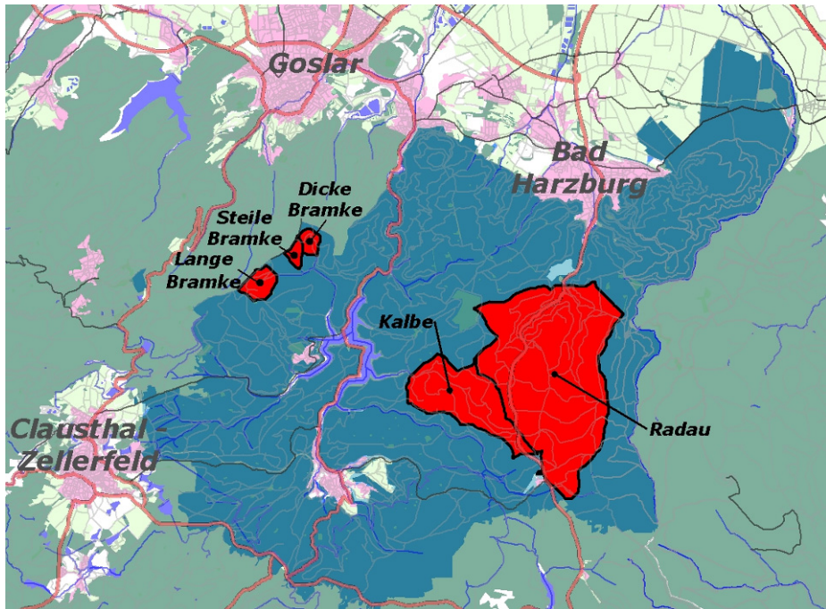
Abbildung 10: Lage ausgewählter Teileinzugsgebiete im Untersuchungsgebiet „Teilbereich Nordharz“. Die Einzugsgebiete der Kalbe und der Radau wurden zur Kalibrierung des hydrologischen Modells herangezogen (s. SUTMÖLLER u. MEESENBURG, in diesem Band).
