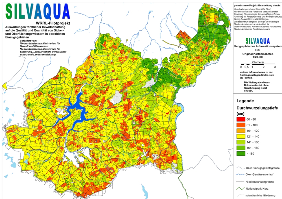
Abbildung 4: Effektive Durchwurzelungstiefe für das Okereinzugsgebiet „Teilbereich Nordharz“
