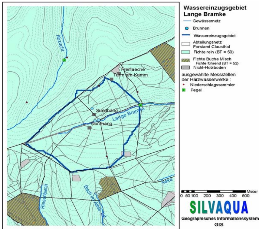
Abbildung 13: Bestandestypen im Teileinzugsgebiet der „Lange Bramke“
