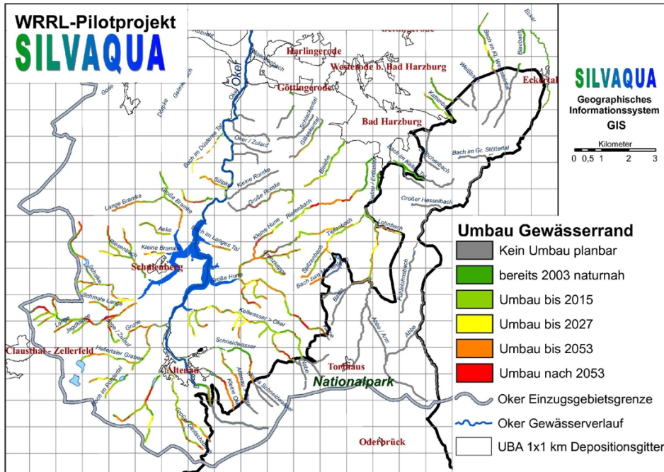
Abbildung 4: Zeitlicher Verlauf eines Gewässerrandstreifenumbaus unter Berücksichtigung der ökonomischen Umtriebszeit im Okereinzugsgebiet „Teilbereich Nordharz“
