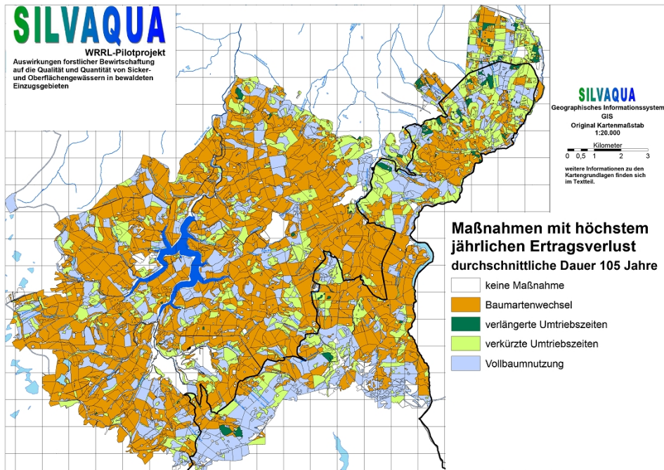
Abbildung 2: Maximale jährliche Ertragsverluste im Untersuchungsgebiet „Nordbarz“ (RÜPING 2009b)
