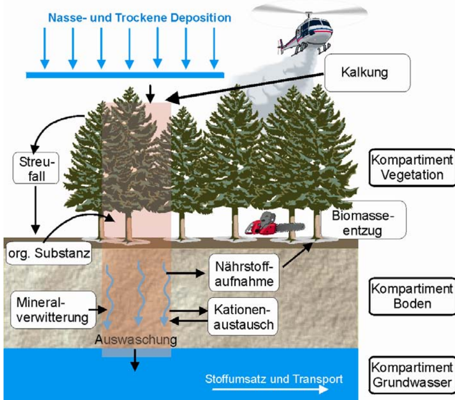
Abbildung 1: Schematische Darstellung der einbezogenen Bilanzgrößen (AHRENDTS et al. 2008)
