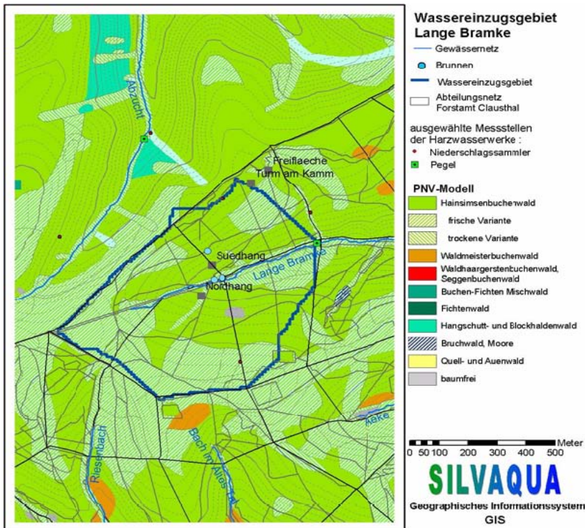
Abbildung 12: Potenziell natürliche Waldgesellschaften im Teileinzugsgebiet der „Langen Bramke“
