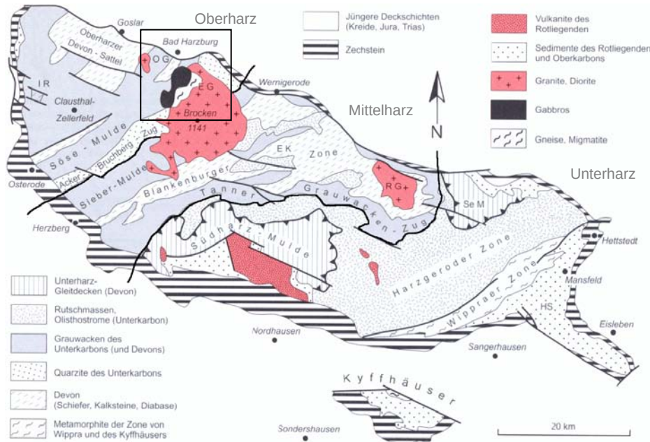
Abbildung 3: Geologische Gliederung des Harzes (n. HENNIGSEN u. KATZUNG 2006, veränd., EG = Eckergneis, EK = Elbingeröder Komplex, HS = Hornburger Sattel, IR = Iberg-Riff, OG = Oker-Granit, RG = Ramberg-Granit, SeM = Selk-Mulde). Der Kasten zeigt die Lage des Teileinzugsgebietes „Nordharz“.
