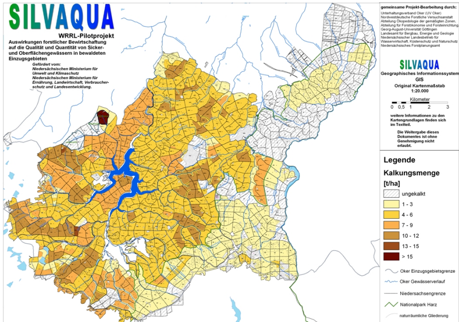
Abbildung 3: Kalkungskataster für das Okereinzugsgebiet „Teilbereich Nordharz“
