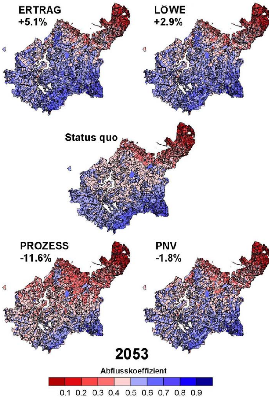
Abbildung 7: Berechnete Abflusskoeffizienten für die Waldentwicklungsszenarien im Zeitfenster 2053
