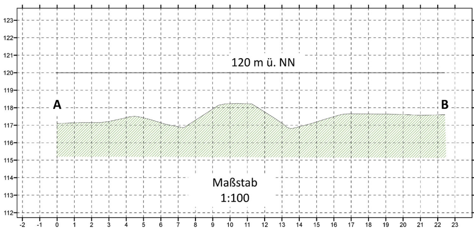
Abb. 5: Querprofil der erhaltenen Wall- und Grabenreste der Sitterhöfer Landwehr (zur Lage des Profils siehe Abb. 3 und 4), erstellt von Dipl.-Ing. Wolfgang REMME, Stadt- und Kreisarchäologie Osnabrück. Alle Angaben in Metern.
