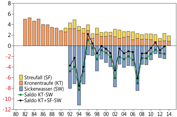
Cadmium-Bilanz Fichte
