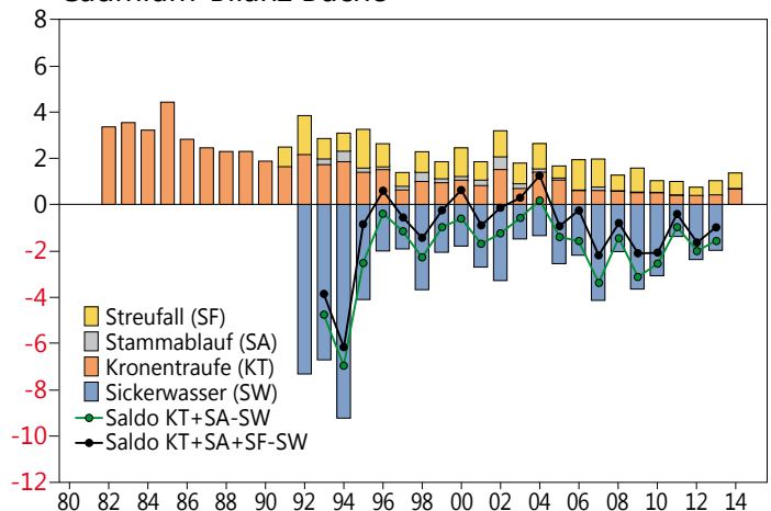
Cadmium-Bilanz Buche
