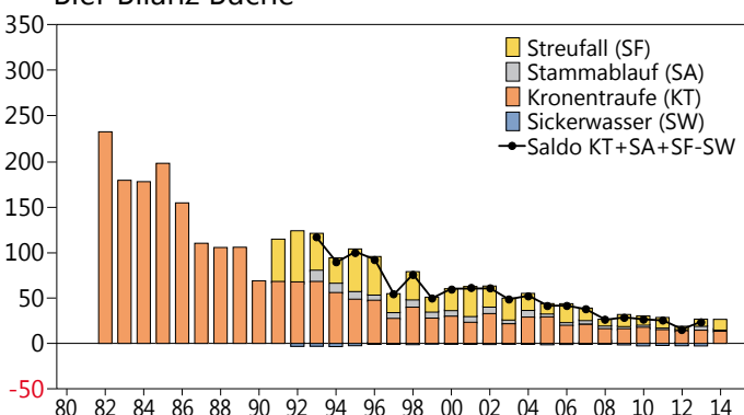
Blei-Bilanz Buche
