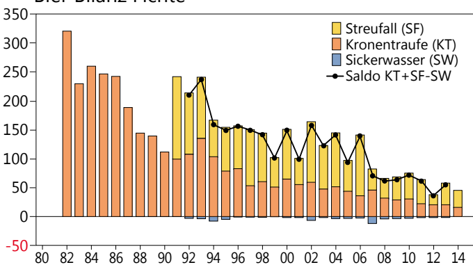
Blei-Bilanz Fichte
