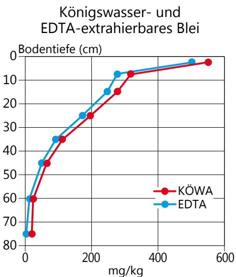
Tiefenprofil der Blei-Gehalte [mg/kg] im Harz (Lange Bramke Kamm) nach unterschiedlichen Extraktionsverfahren
