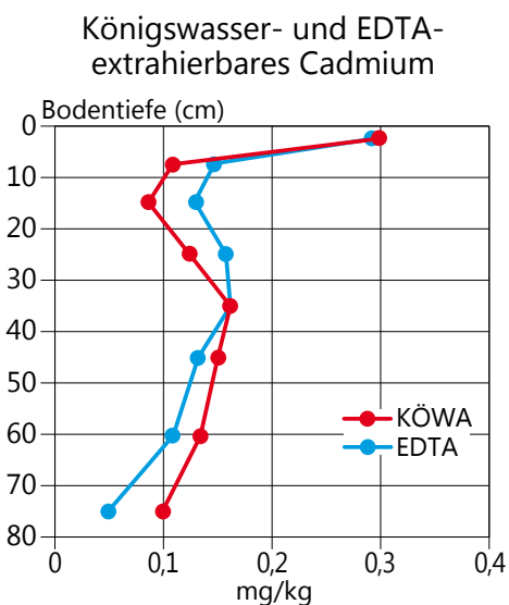
Tiefenprofil der Cadmium-Gehalte [mg/kg] im Harz (Lange Bramke Kamm) nach unterschiedlichen Extraktionsverfahren
