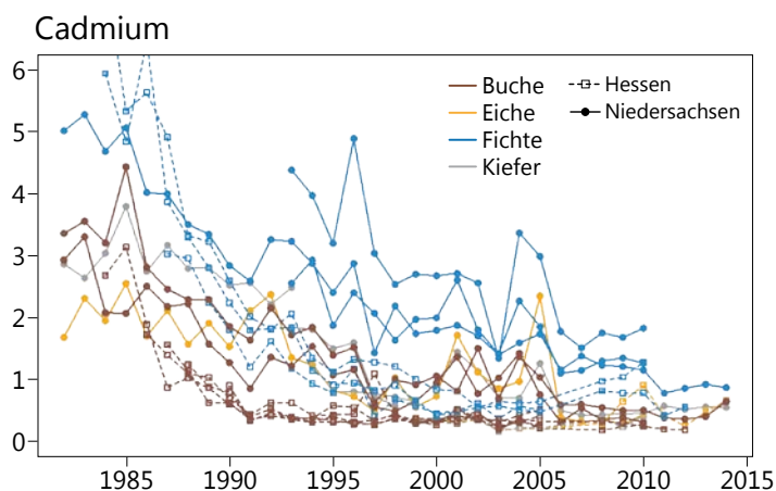
Jährliche Cadmium-Einträge (Gramm je Hektar) mit der Kronentraufe für 20 Flächen des Intensiven Waldmonitorings in Hessen und Niedersachsen von 1982-2014
