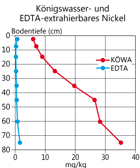
Tiefenprofil der Nickel-Gehalte [mg/kg] im Harz (Lange Bramke Kamm) nach unterschiedlichen Extraktionsverfahren
