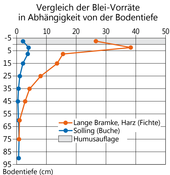
Tiefenprofil der Blei-Vorräte (kg je Hektar und cm) in der Lange Bramke, Harz (Fichte) und im Solling (Buche)
