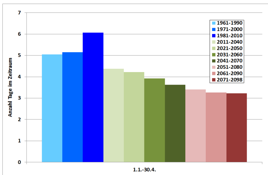
Abbildung 2.9: Anzahl der Tage mit Wechselfrost im Zeitraum 1.1.-30.4., Deutschlandmittel für 30-jährige Zeiträume in Vergangenheit und Zukunft
